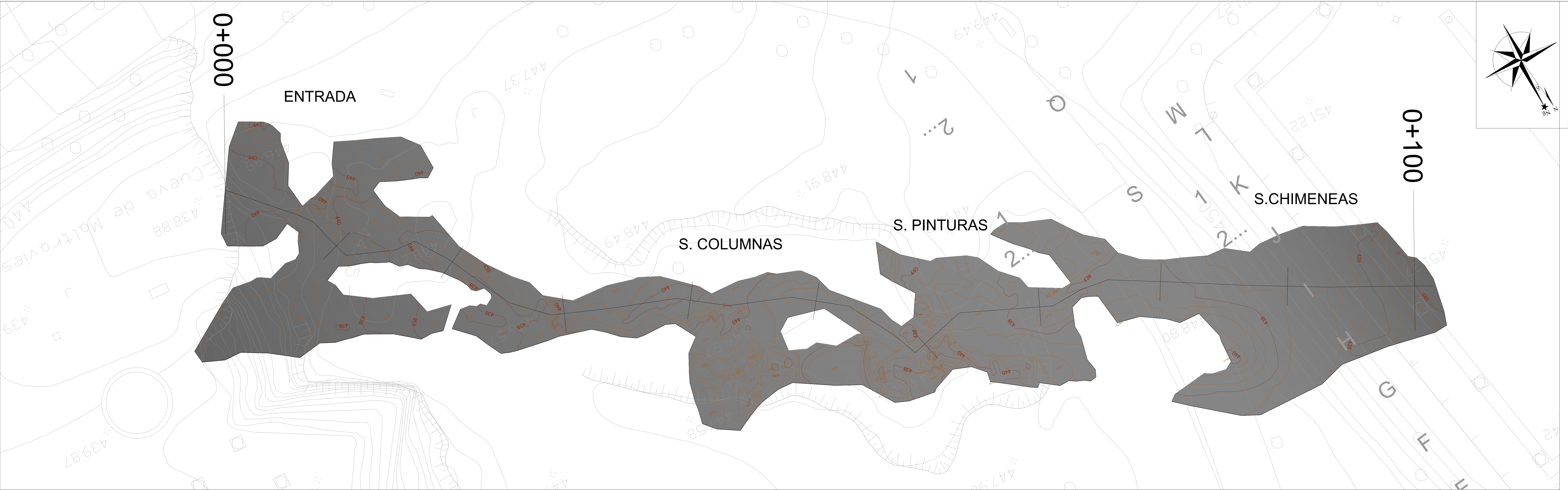
PLANTA E: 1/300
